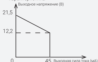
Выходная характеристика
