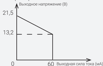
Выходная характеристика
