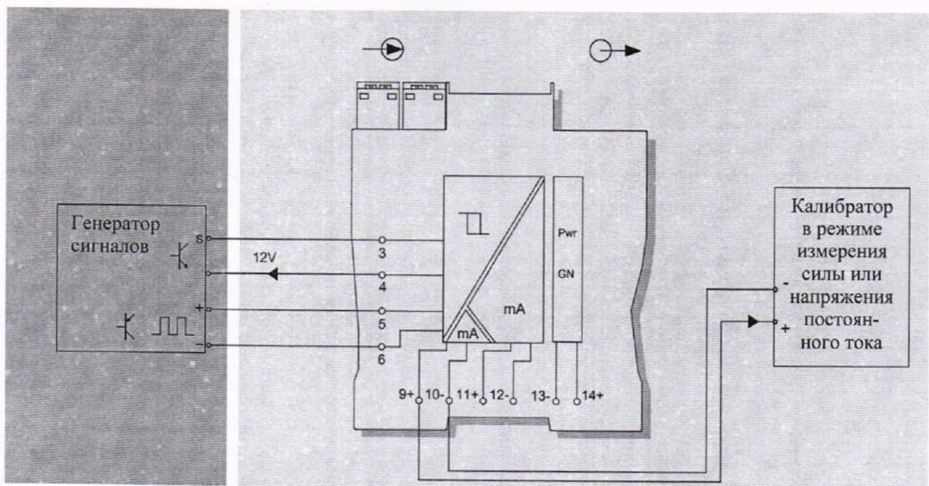
Рис. А.39 Схема подключения барьеров искрозащиты BIS-EXA-N6*A1P1, BIS-EXA-N6*A1P2
