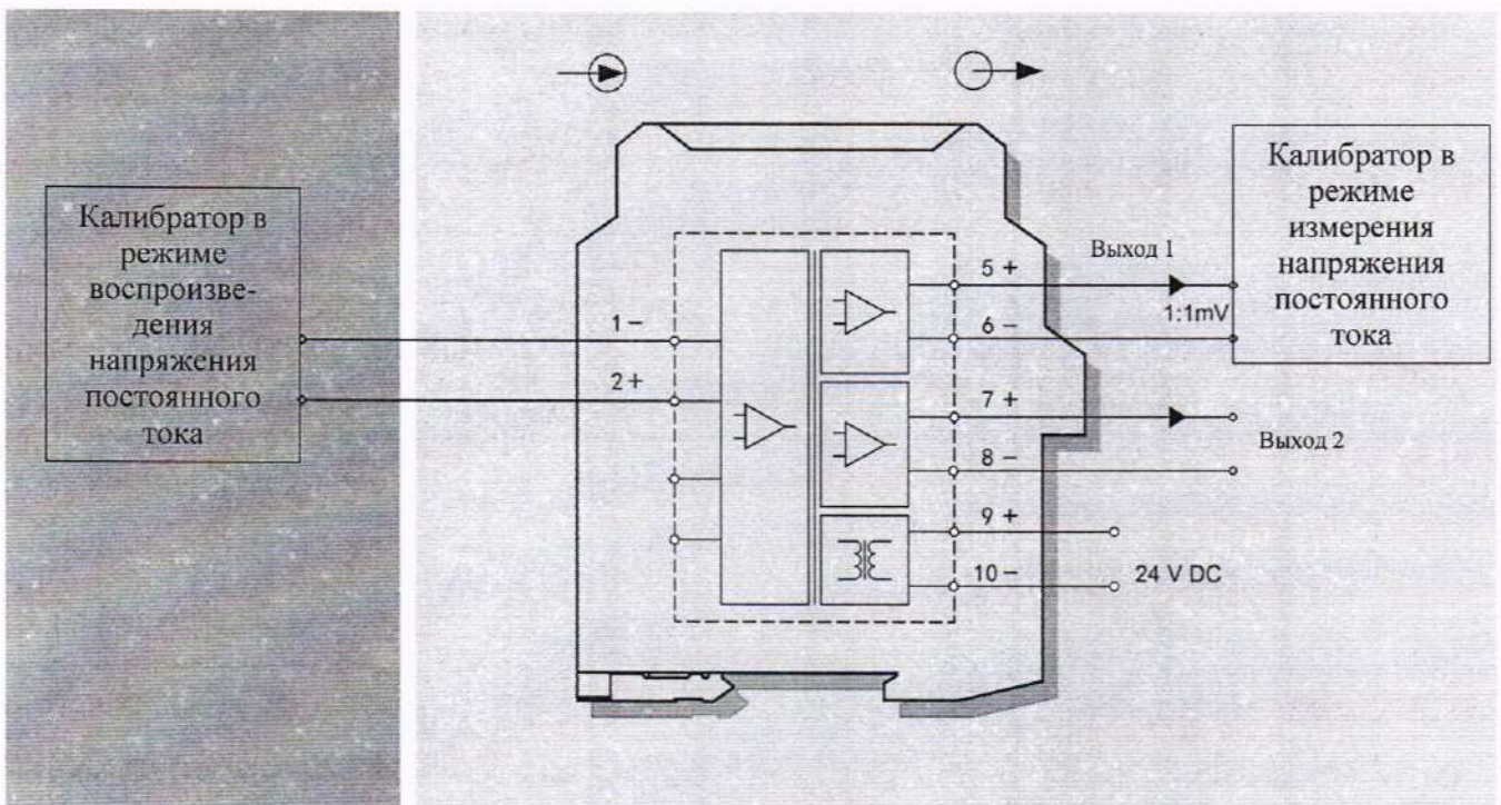
Рис. А.6 Схема подключения барьеров искрозащиты BIS-EXA-C17*, BIS-EXA-CM17*
