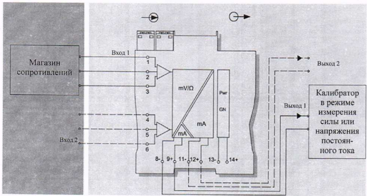
Рис. А.31 Схема подключения барьеров искрозащиты BIS-EXA-H2**, BIS-EXA-H2D** и BIS-EXA-H0**, BIS-EXA-H0D** в режиме преобразования сигналов от термосопротивлений
