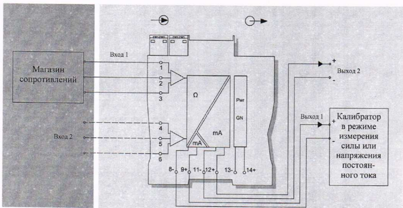
Рис. А.40 Схема подключения барьеров искрозащиты BIS-EXA-N9**, BIS-EXA-N9D**
