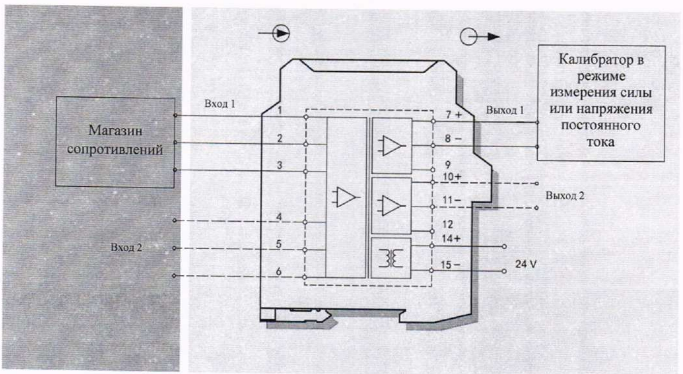
Рис. А.2 Схема подключения барьеров искрозащиты ВИС-ЕХА-С0*Н, ВИС-ЕХА-С0**Н, ВИС-ЕХА-С0D**, ВИС-ЕХА-С2D**, ВИС-ЕХА-К01 в режиме преобразования сигналов от термосопротивлений
