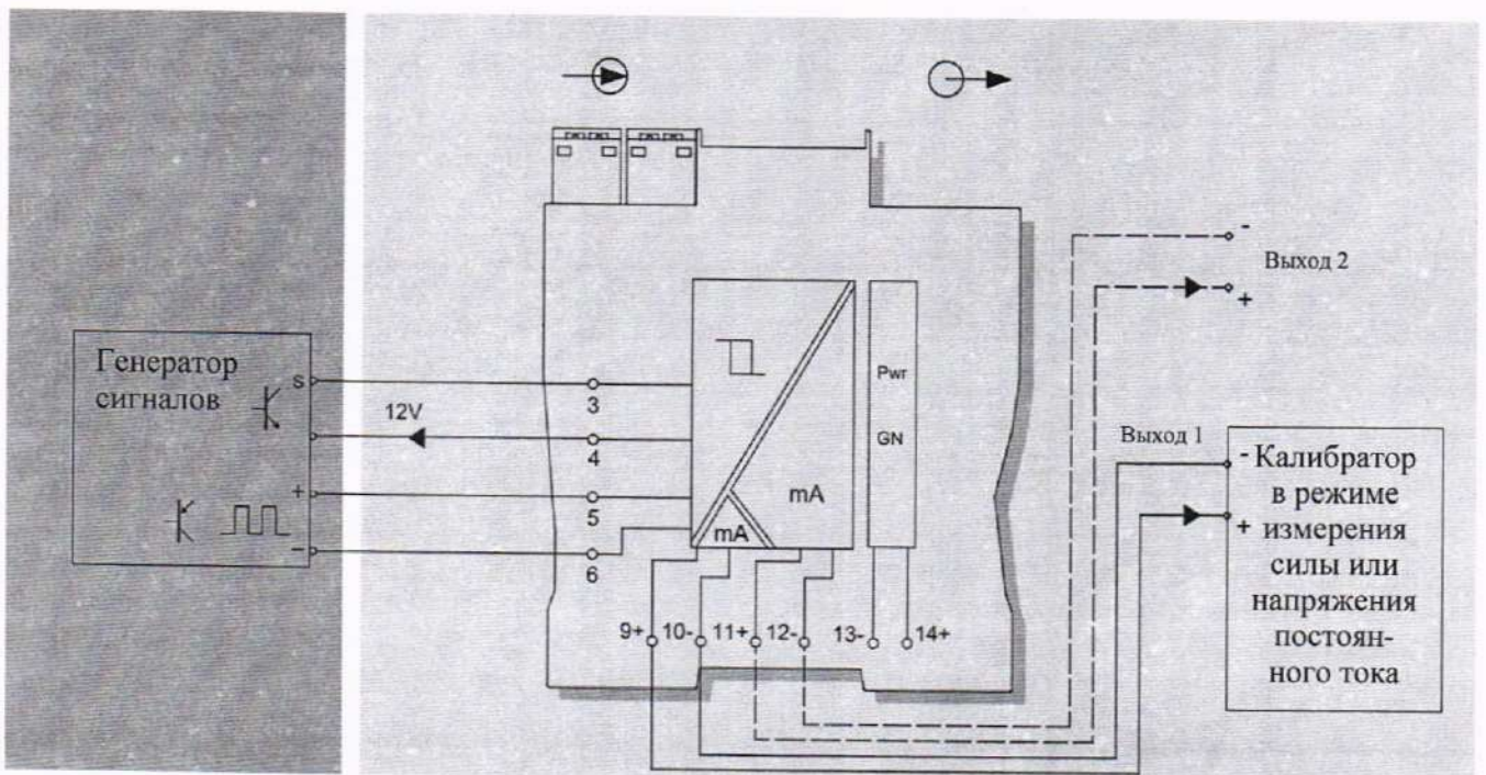
Рис. А.38 Схема подключения барьеров искрозащиты BIS-EXA-H6*P1, BIS-EXA-H6**P1, BIS-EXA-H6*P2, BIS-EXA-H6**P2
