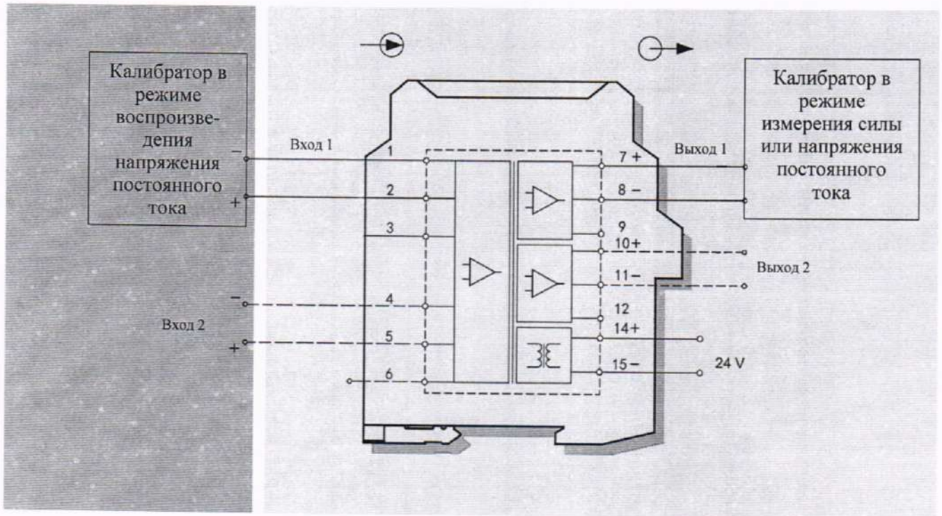
Рис. А.1 Схема подключения барьеров искрозащиты ВИС-ЕХА-С0*Н, ВИС-ЕХА-С0**Н, ВИС-ЕХА-С0D**, ВИС-ЕХА-К01, ВИС-ЕХА-С1*Н, ВИС-ЕХА-С1**Н, ВИС-ЕХА-С1D** в режиме преобразования сигналов от термопар
